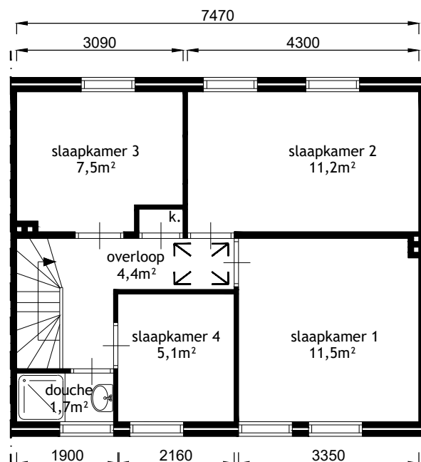
verdieping
