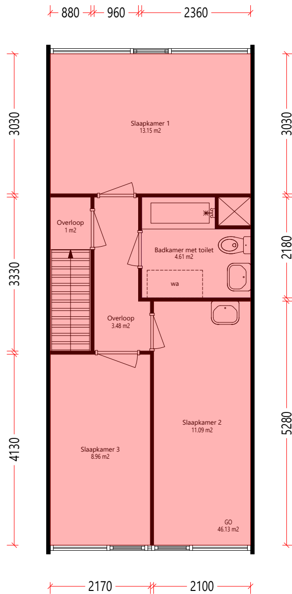
Verdieping_2e
