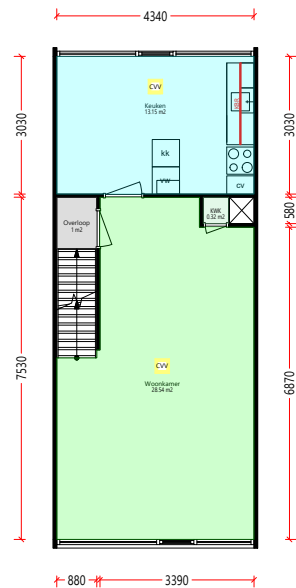
Verdieping_1e
