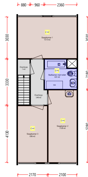
Verdieping_2e
