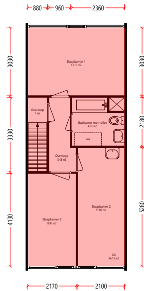
Verdieping_2e
