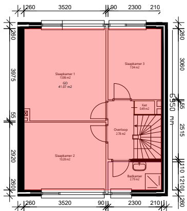
Verdieping_1e
