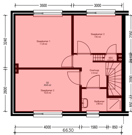
Verdieping_1e
