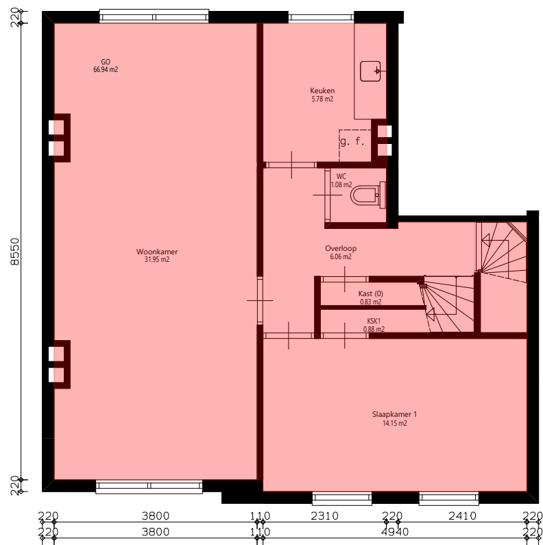
Verdieping_1e
